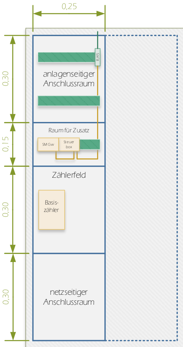
Abbildung 1 – Zäblerschrank eHz
