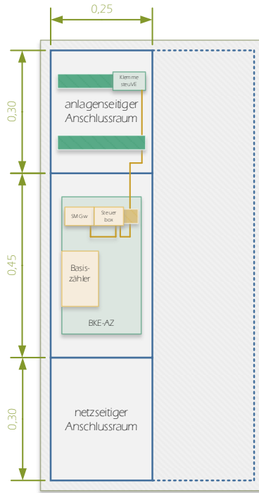
Abbildung 4 – Zählerschrank 3.Hz
