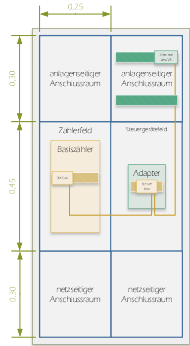
Abbildung 5 – Zählerschrank 3.Hz inkl. Steuergerätefeld
