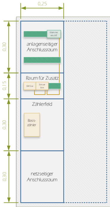
Abbildung 3 – Zählerschrank eHz
