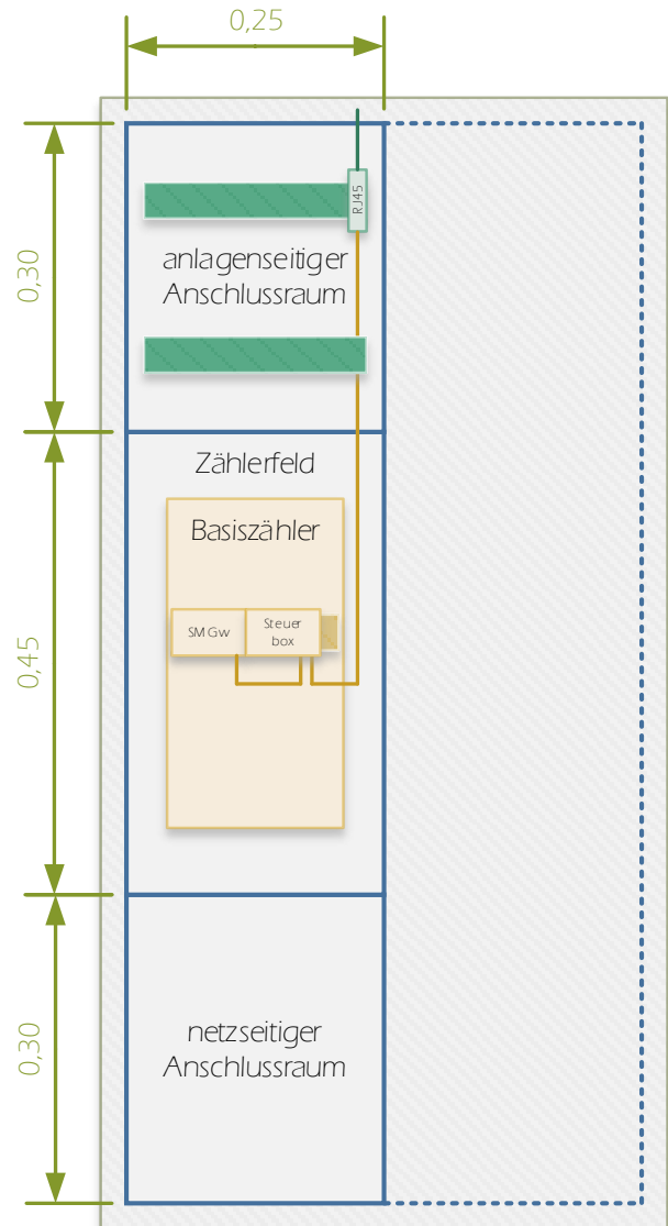
Abbildung 2 – Zäblerschrank 3.Hz
